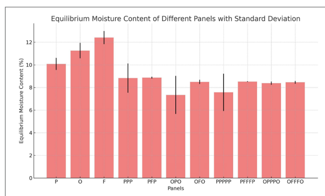
Fig. 8. Equilibrium moisture content of CLTs
